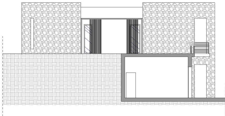
PROSPETTO 2-2
