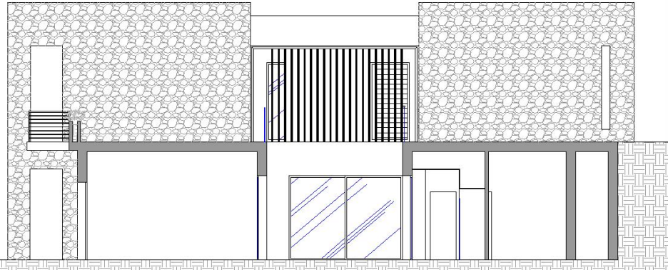
PROSPETTO 1-1
