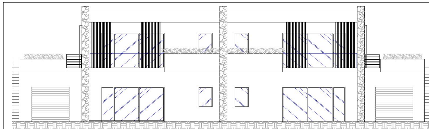
PROSPETTO 3-3
