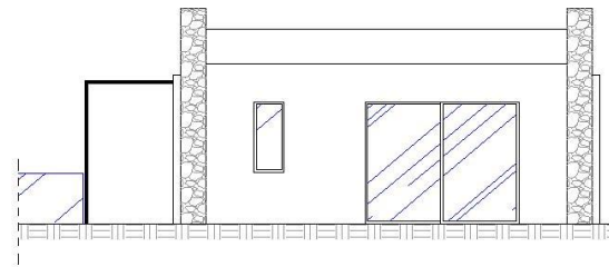
PROSPETTO 4-4
