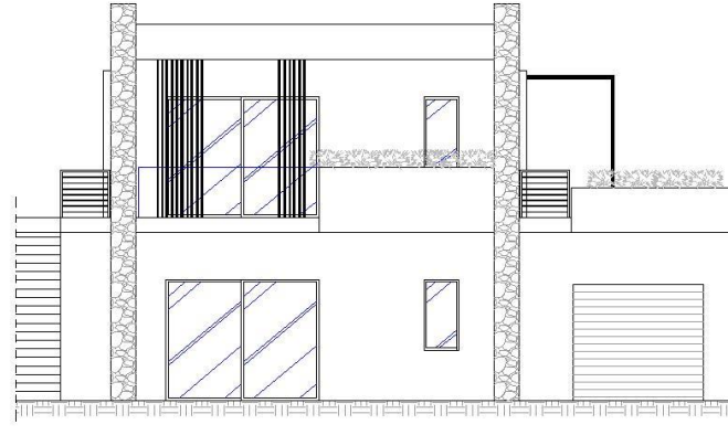
PROSPETTO 3-3
