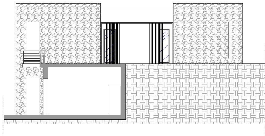
PROSPETTO 1-1
