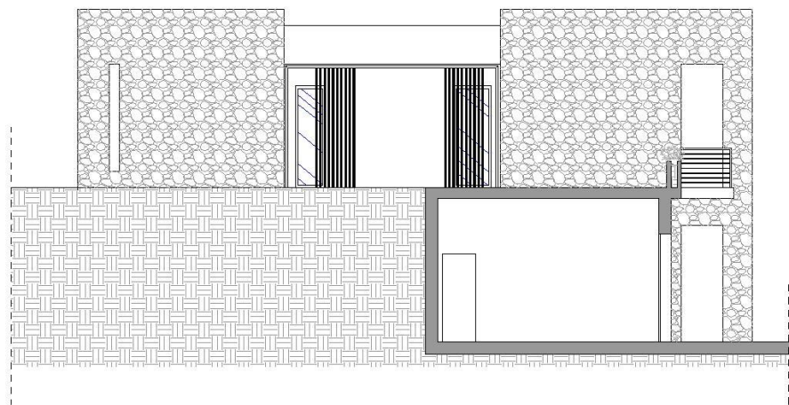
PROSPETTO 2-2
