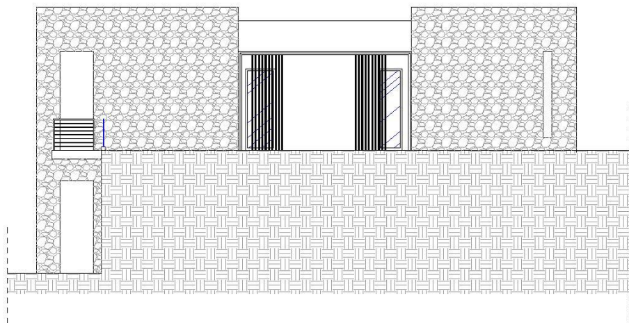
PROSPETTO 1-1
