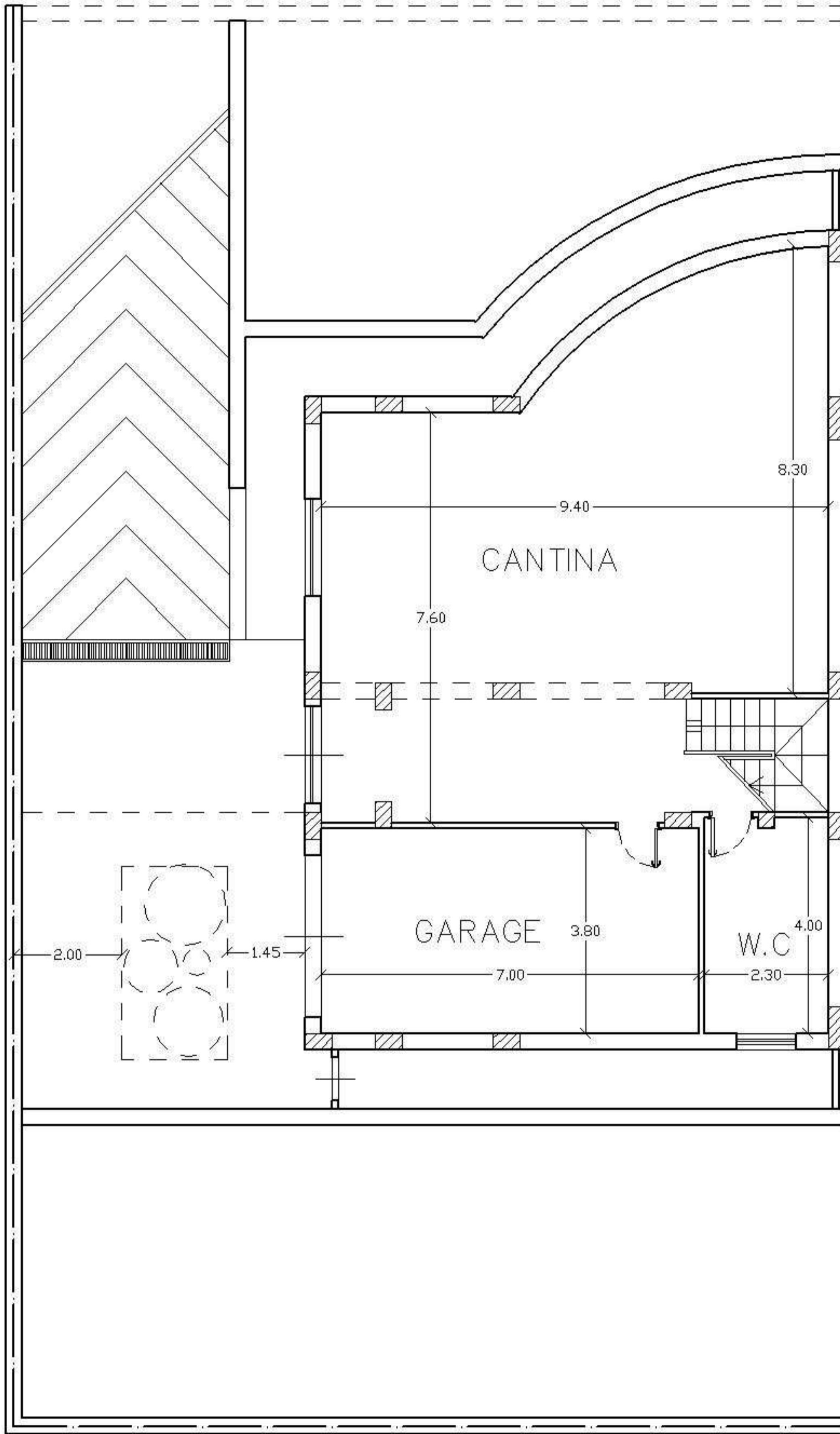
PIANTA PIANO INTERRATO
